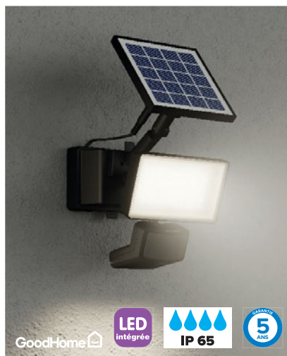
Projecteur à détection Davern 6 W 400 lumens Réf. 5059340191256. Existe en 800 ou en 2 x 800 lumens (1) .
